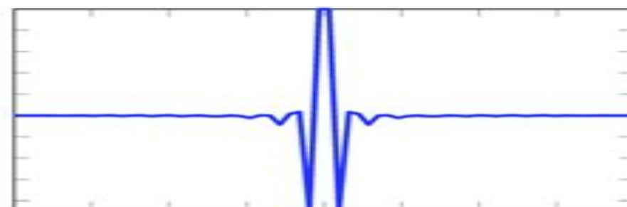
(d) Spline Wavelet
