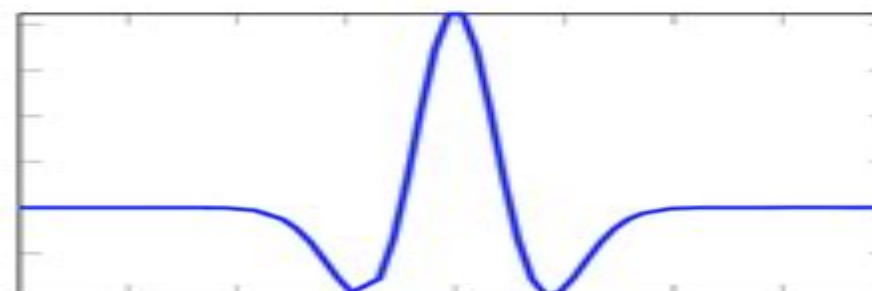
(e) Mexican Hat Wavelet
