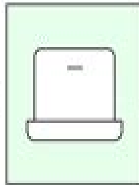
XML Parser
