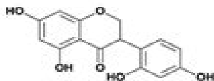
Dalbergioidin (8)
