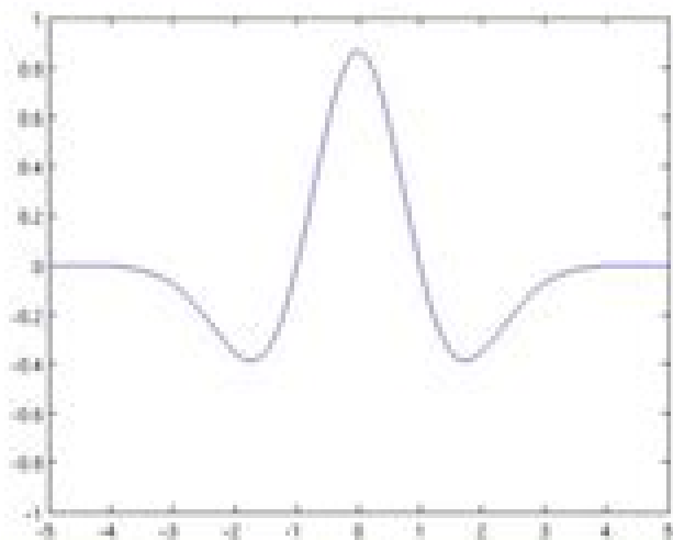
Mexican hat wavelet
