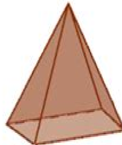
Pyramid
