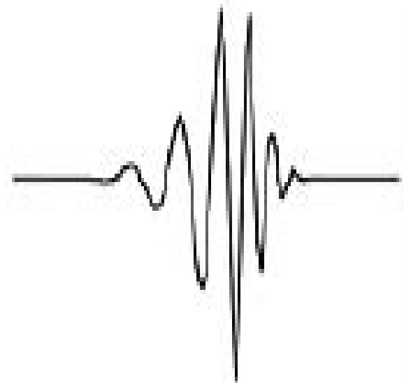
Daubechies 20
