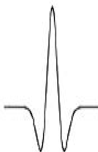
Mexican Hat
